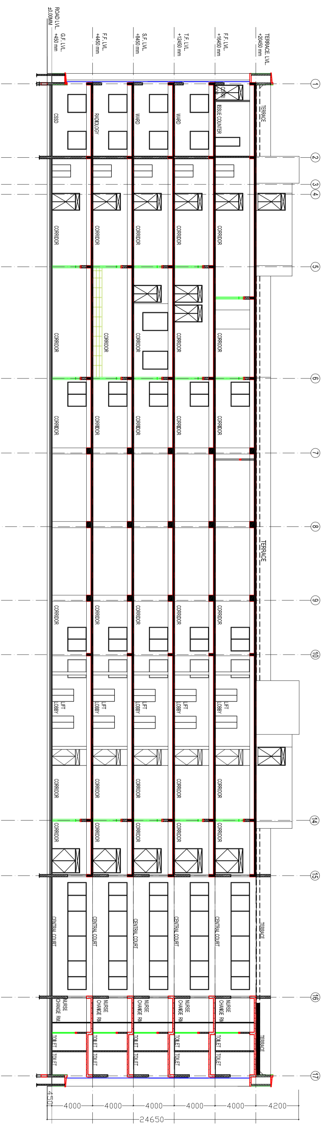
SECTION A-A
